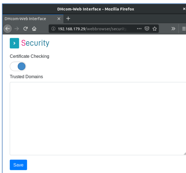
Abbildung 16 - Webbrowser Security
